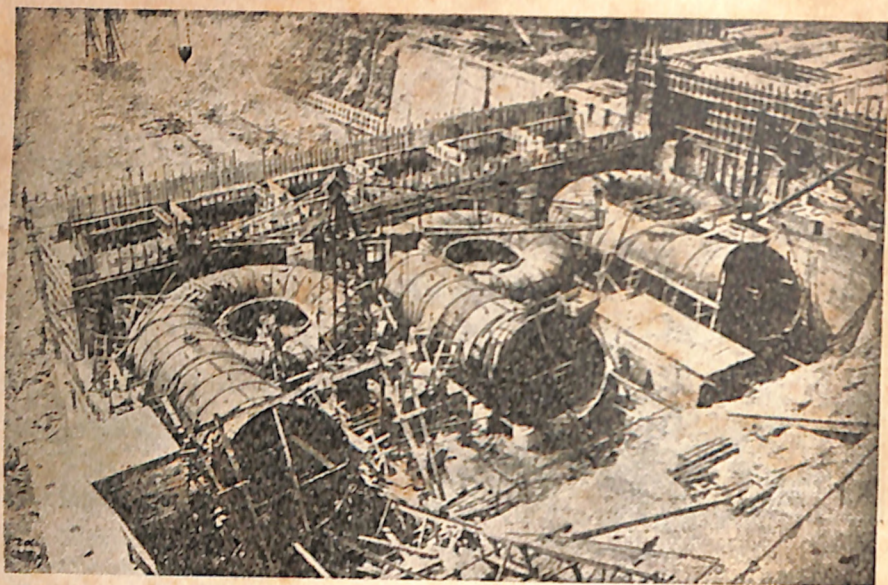
Instalação das turbinas duma usina elétrica moderna nos Estados-Unidos.
